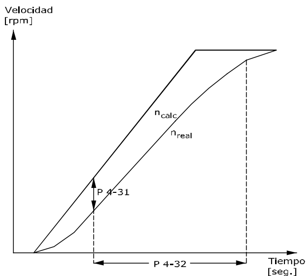
130BA221.10 Ilustración 4.8 Error de velocidad en realim. del motor
