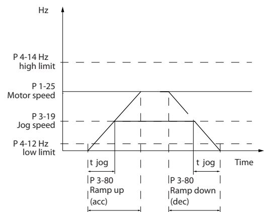
Ilustración 4.6 Tiempo rampa veloc. fija
