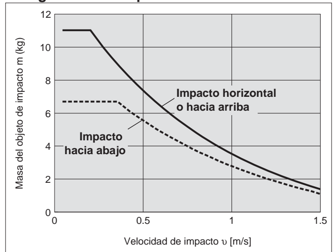
Energía absorbida por RJ1007H
