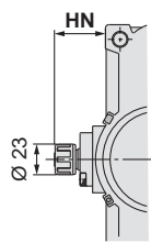
Mecanismo de bloqueo en final de carrera (Modelo de desbloqueo manual)
