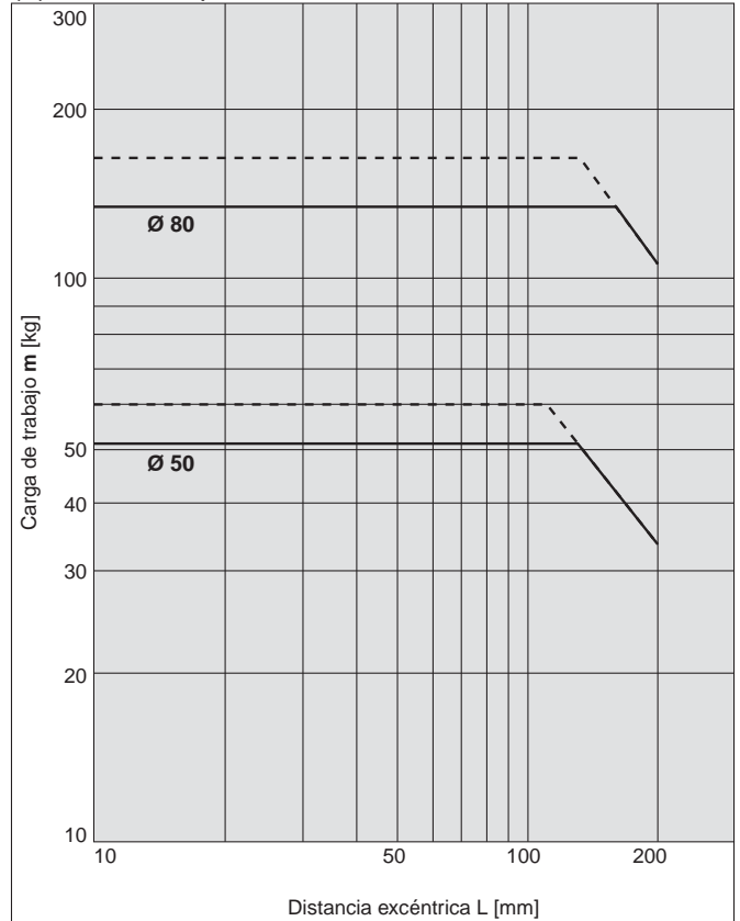
(2) Carrera superior a 50 mm, V = 200 mm/s o menos
