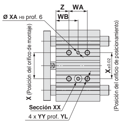
Vista inferior
