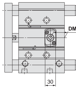
Con bloqueo en extremo posterior
