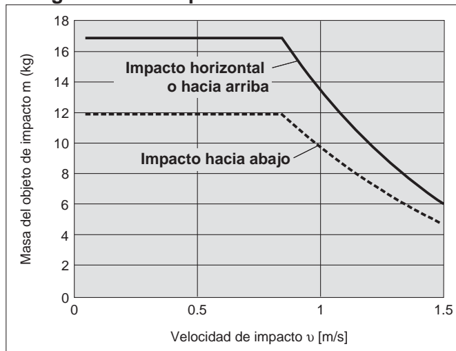
Energía absorbida por RJ1412H
