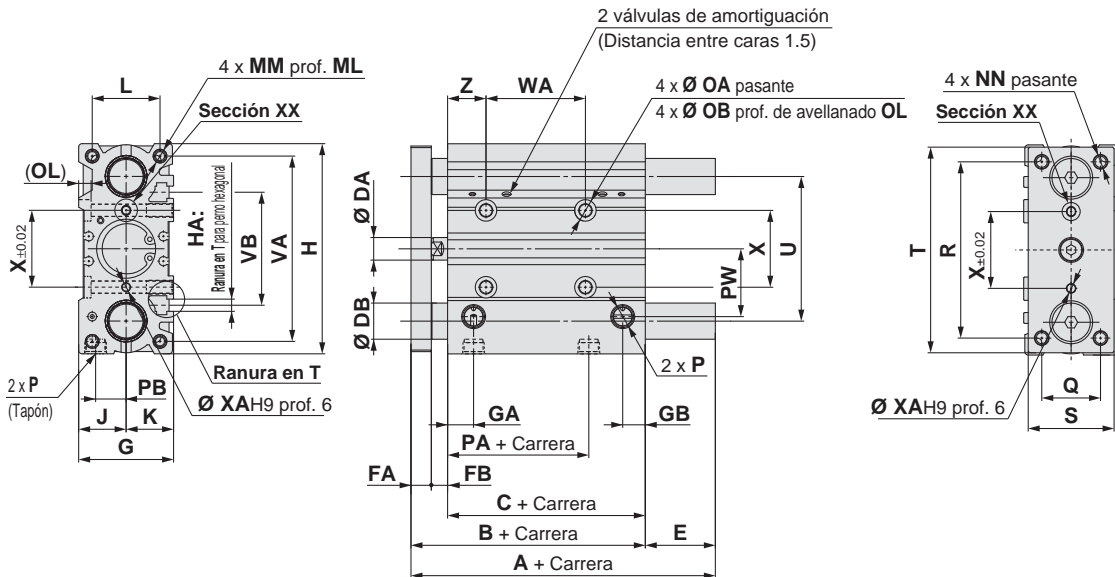
Vista inferior
