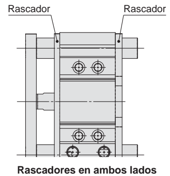
Rascadores en ambos lados
