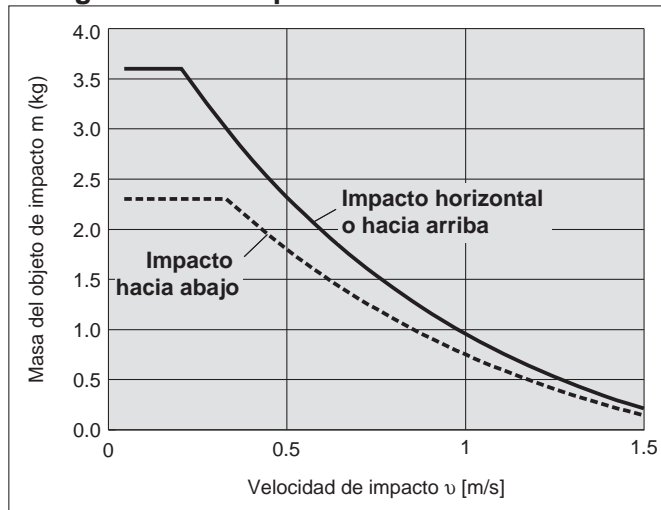
Energía absorbida por RJ1412H
