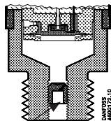
Amortiguador de pulsos
